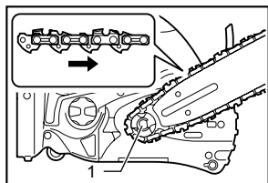
1. Sprocket
